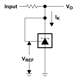
简化原理图
