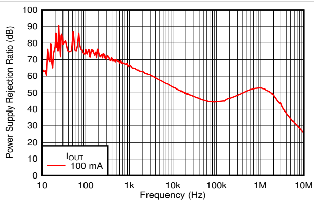
图 9-4. PSRR Performance
