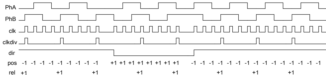
图 20-3. 正交编码器和速度预分频器的操作
