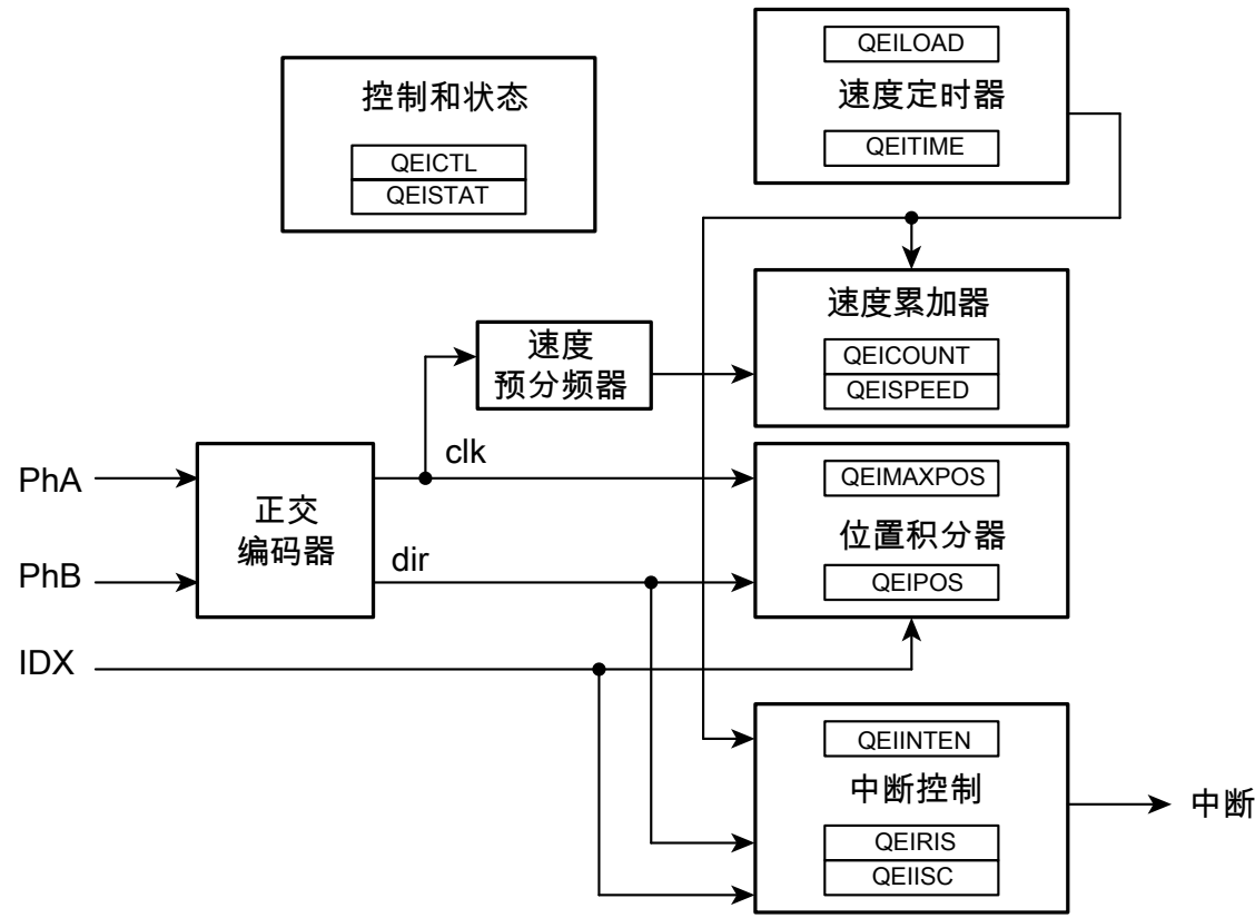
图 20-1. QEI结构图
