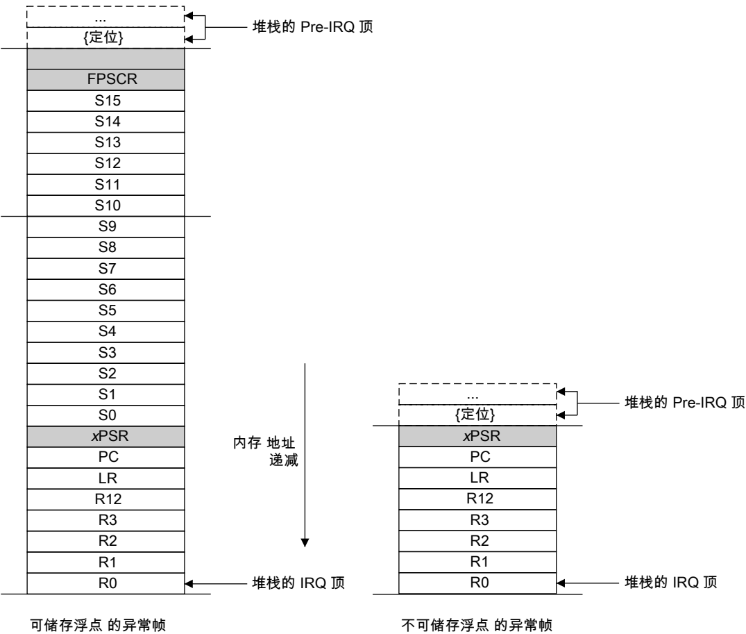
图 2-7. 异常堆栈框
