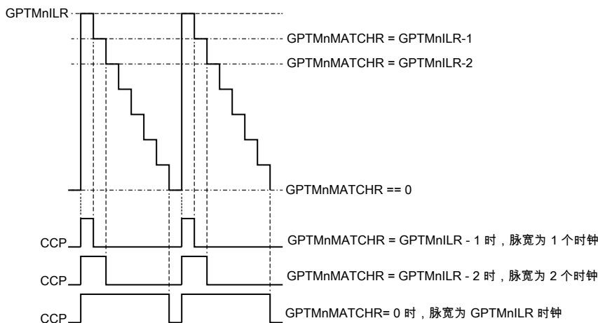
图 11-8. CCP 输出，GPTMTnILR &gt; GPTMTnMATCHR
