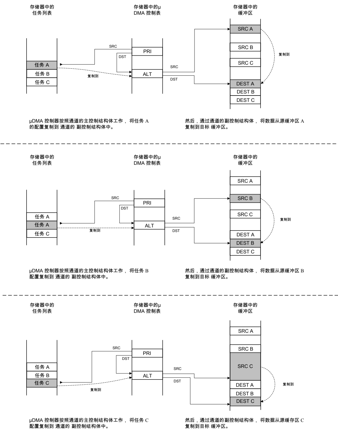
图 9-4. 存储器散聚模式：μDMA 复制序列
