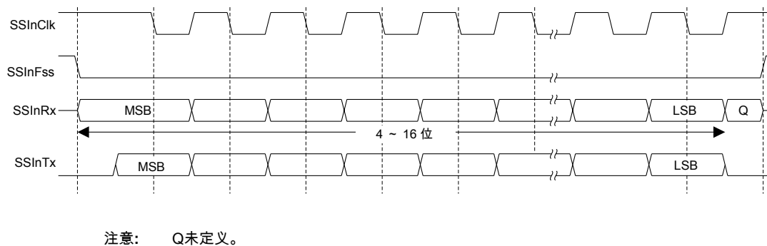
图 15-8. SPO = 1 和 SPH = 0 时的飞思卡尔 SSI 帧格式 ( 连续传输 )
