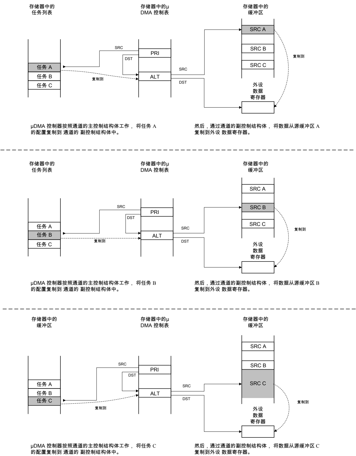
图 8-6. 外设散聚模式：μDMA 复制序列
