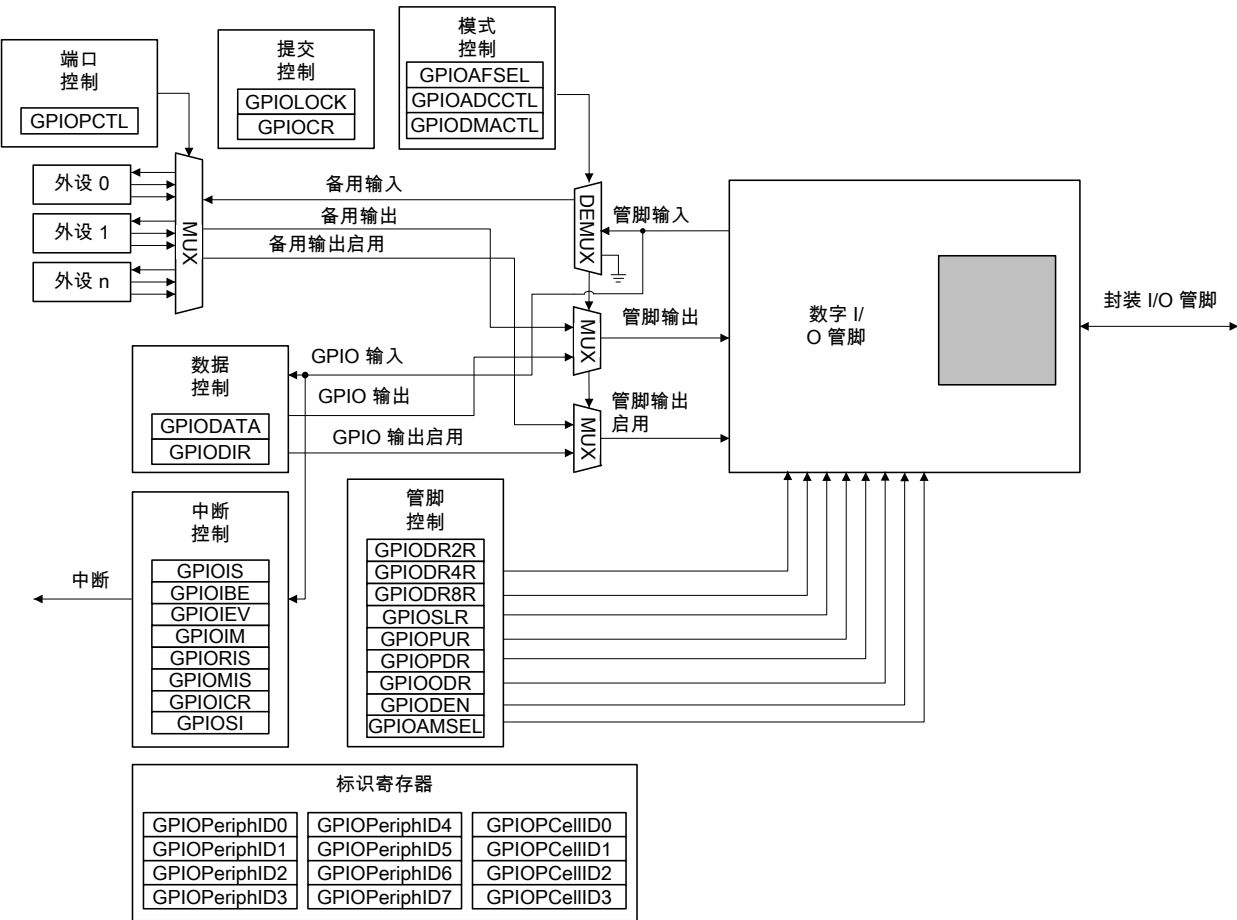
图 9-1. 数字 I/O 口
