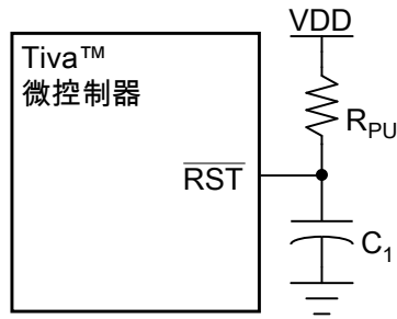
图 5-2. 延长上电复位时间的外部电路
