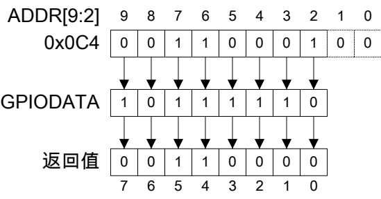
图 9-4. GPIODATA 读实例
