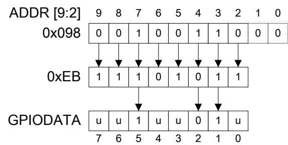
图 9-3. GPIODATA 写实例
