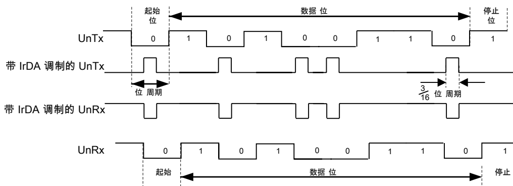
图 13-3. IrDA 数据调制
