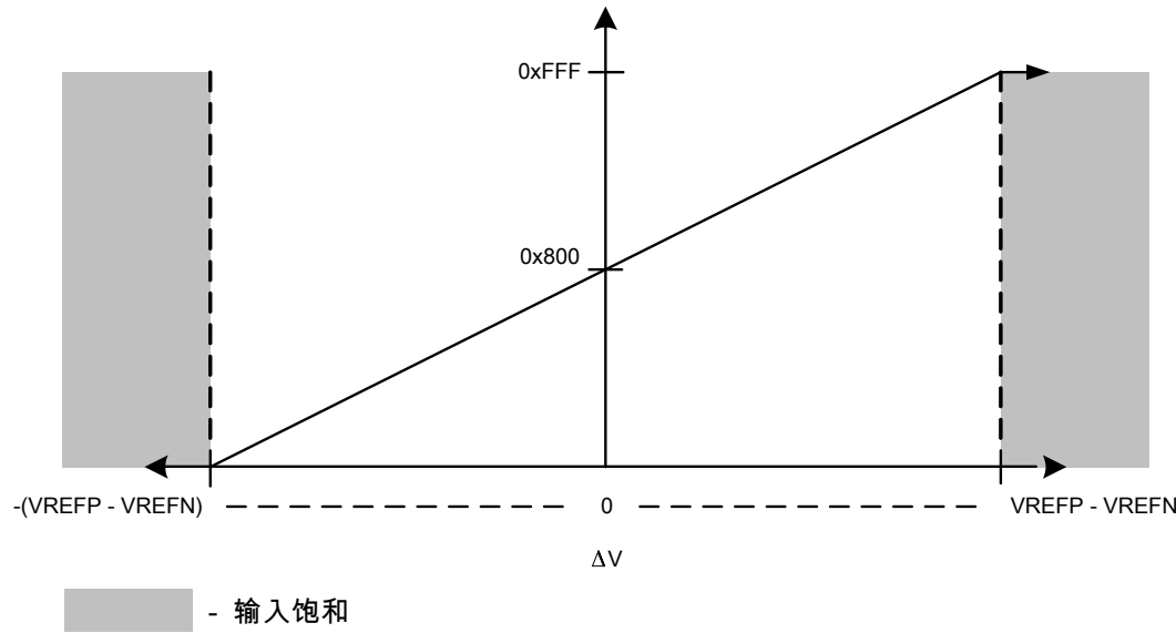
图 12-10. 差分电压表达式
