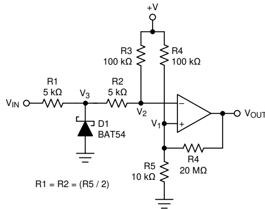
图 8-17. 过零检测器
