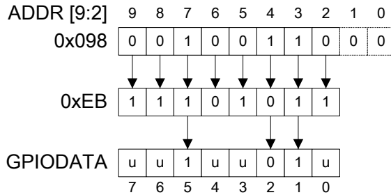
图 9-3. GPIODATA 写实例
