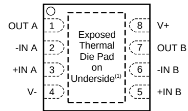
TLV9062 DSG 封装 带有外露散热焊盘的 8 引脚 WSON 封装 俯视图
