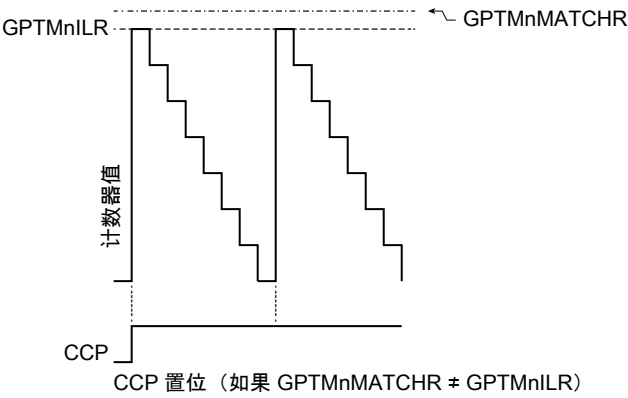
图 11-6. CCP 输出，GPTMTnMATCHR > GPTMTnILR
