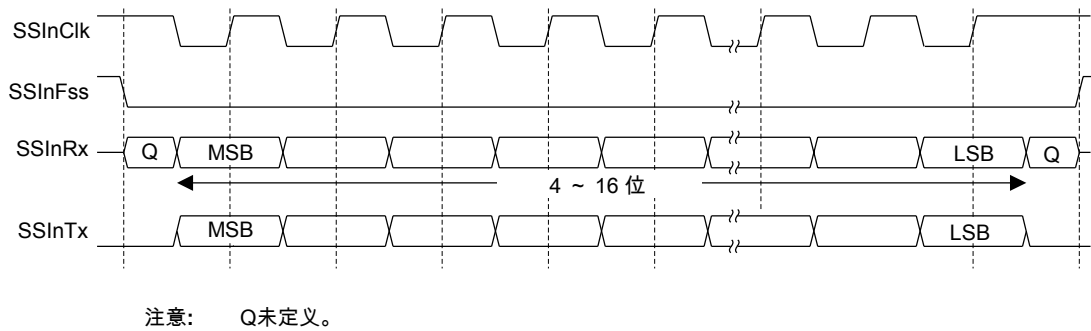
图 15-9. SPO = 1、SPH = 1 时的飞思卡尔 SPI 帧格式
