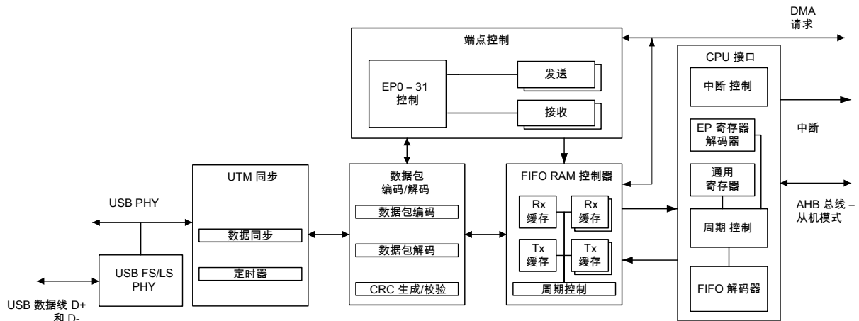
图 18-1. USB 模块结构图
