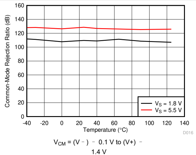
图 7-16. DC CMRR vs Temperature
