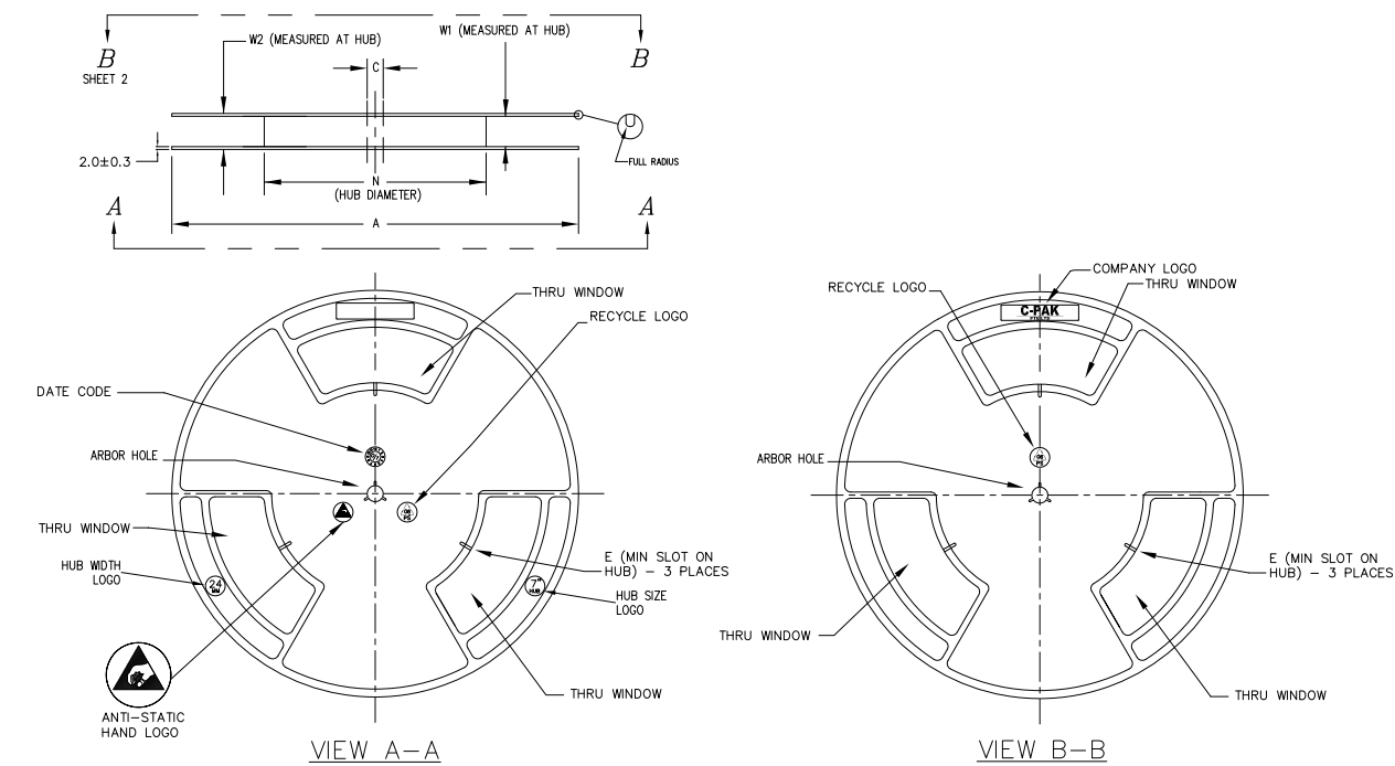
图 A-4. 100 管脚 LQFP PZ 封装塑料圆盘
