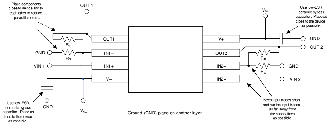
图 11-2. Layout Example
