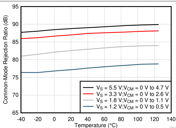
图 7-20. DC CMRR vs Temperature
