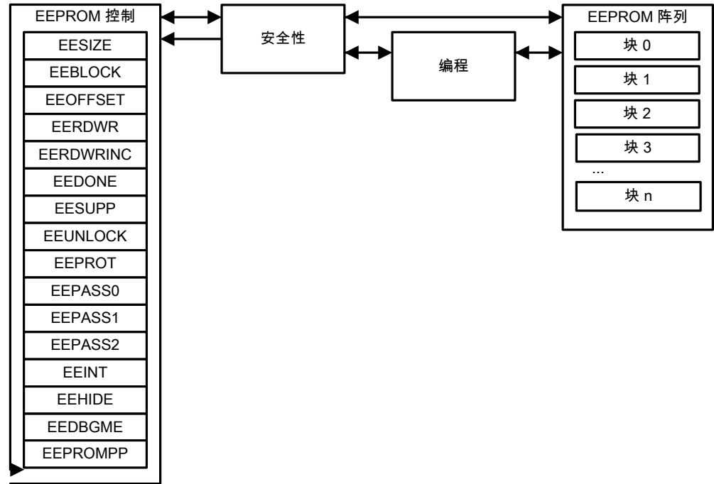
图 7-2. EEPROM 结构图
