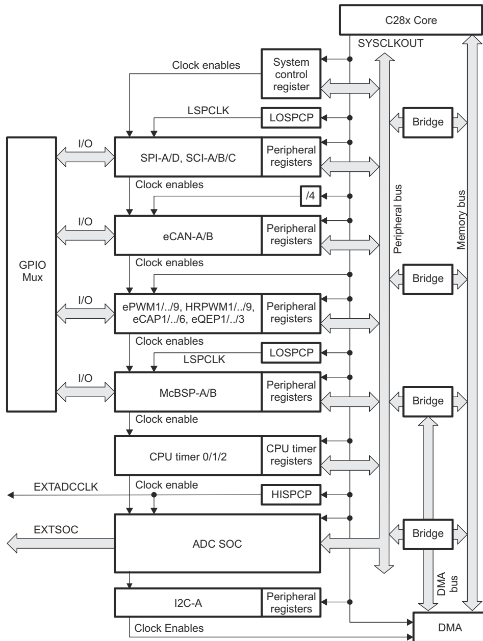
图 8-27. Clock and Reset Domains
