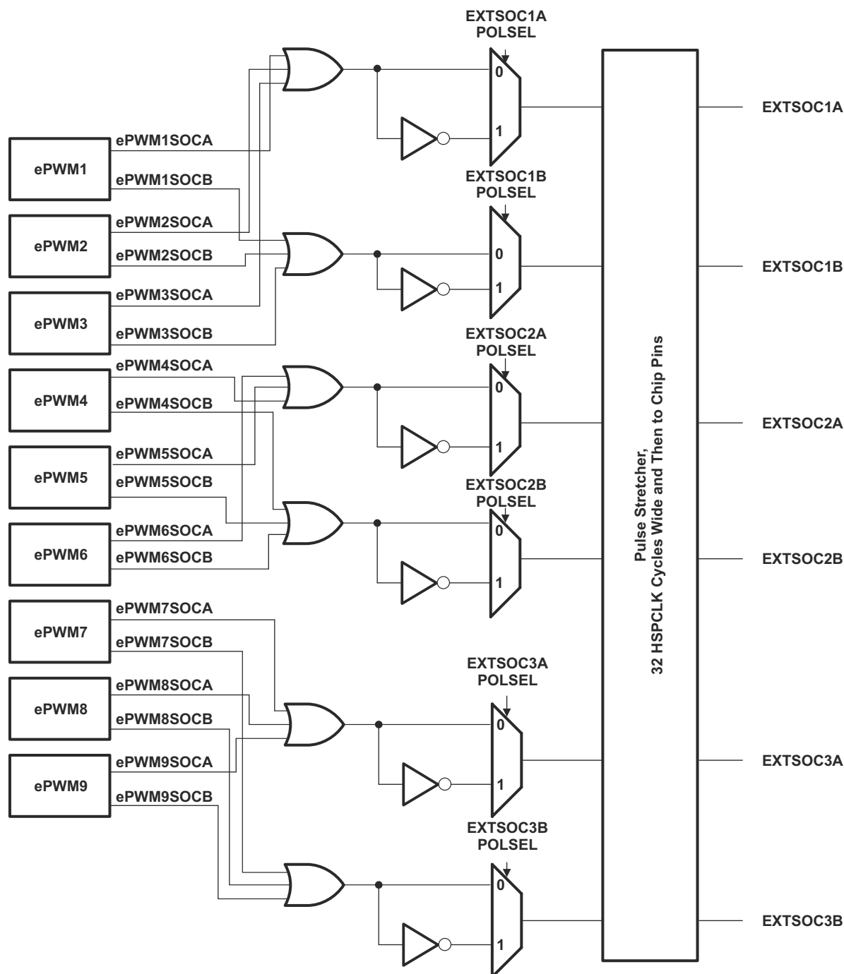
图 8-8. External ADC Interface
