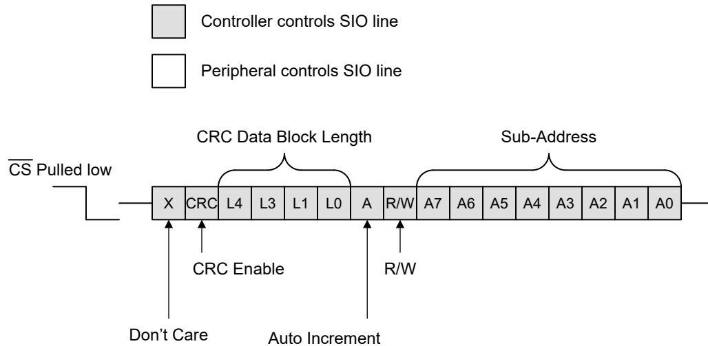
图 8-10. TMP126 Command Word
