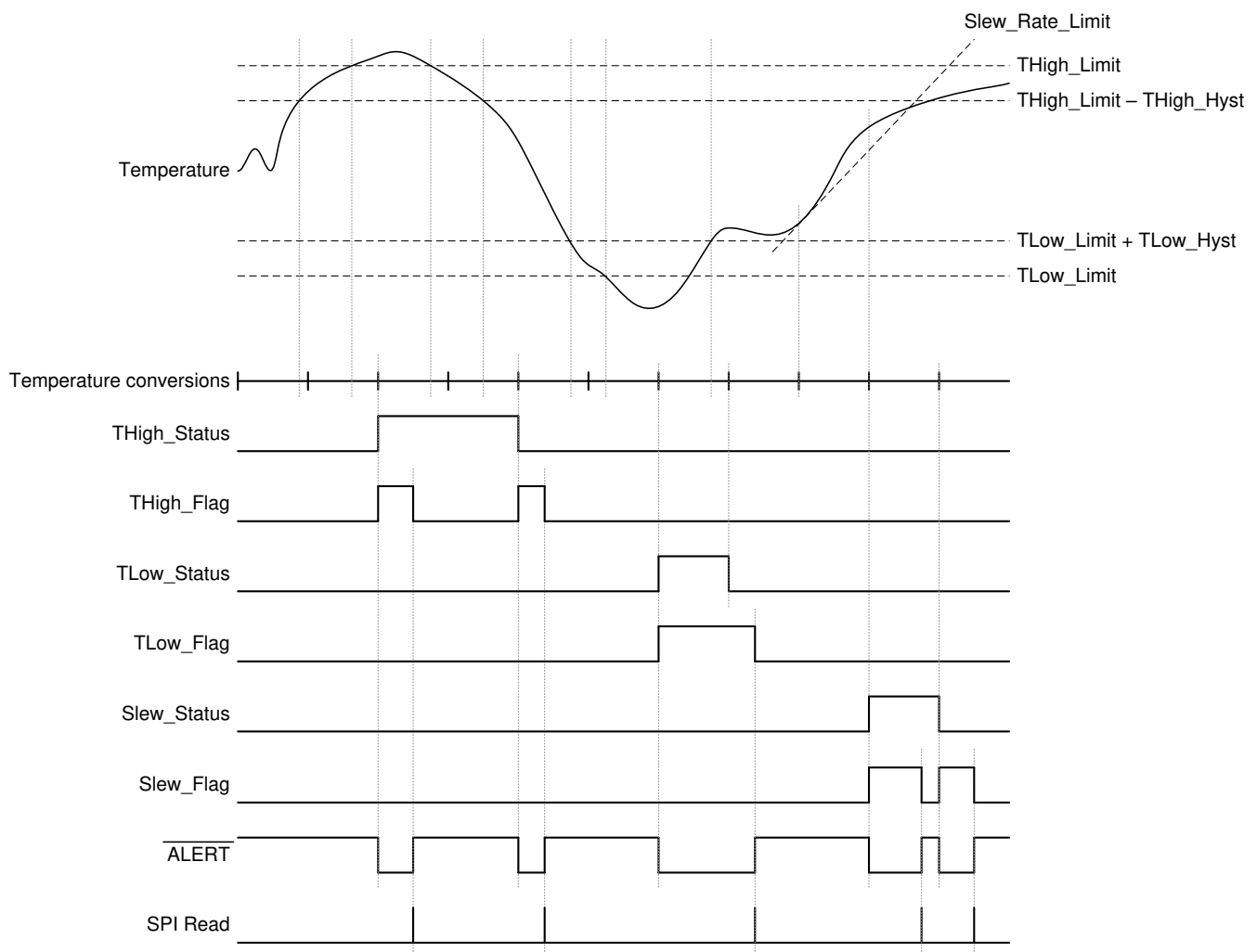
图 8-7. Interrupt Mode Diagram
