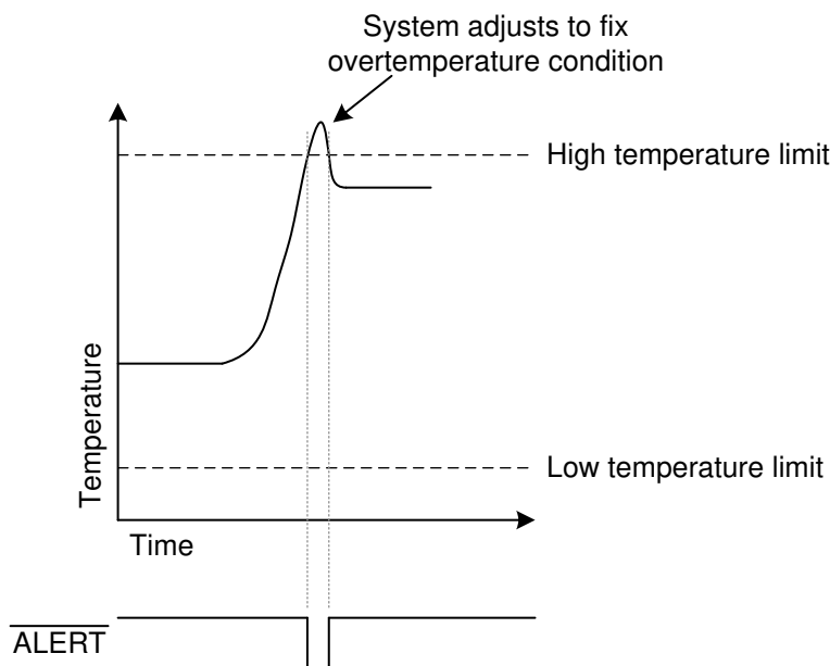
图 8-1. Temperature Limit Alert
