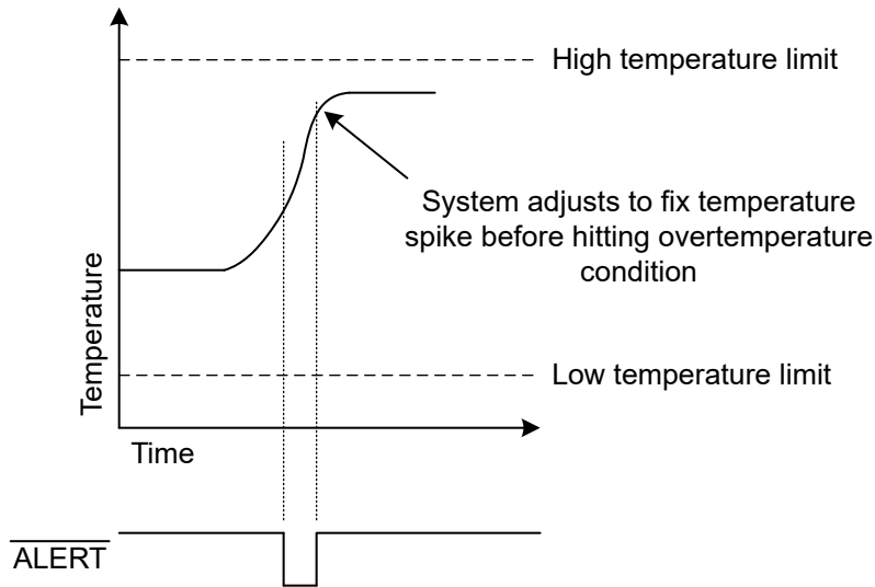
图 8-2. Slew Rate Warning
