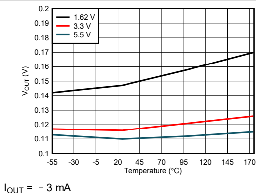
图 7-9. ALERT Output vs Temperature
