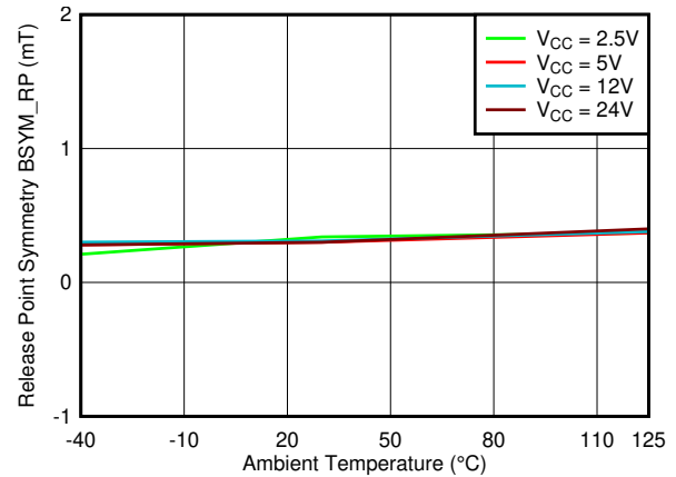
图 7-32. B_{SYM\_RP(ZY)} vs. Temperature
