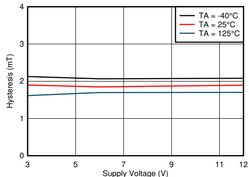
图 7-6. Hysteresis vs V_{CC}
