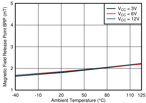
图 7-3. B_{RP} vs Temperature
