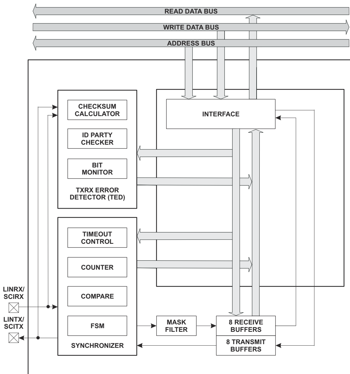
图 8-34. LIN Block Diagram
