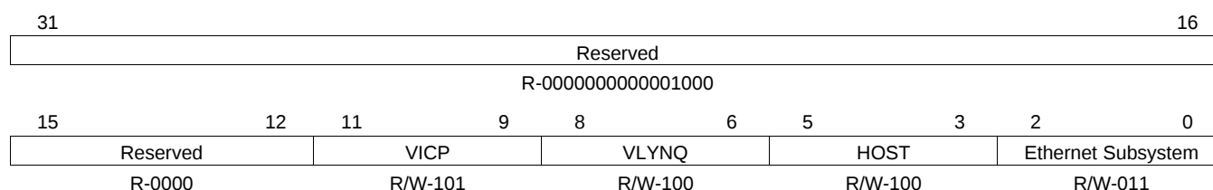
Figure 3-4. Priority Allocation Register (PRI_ALLOC)
