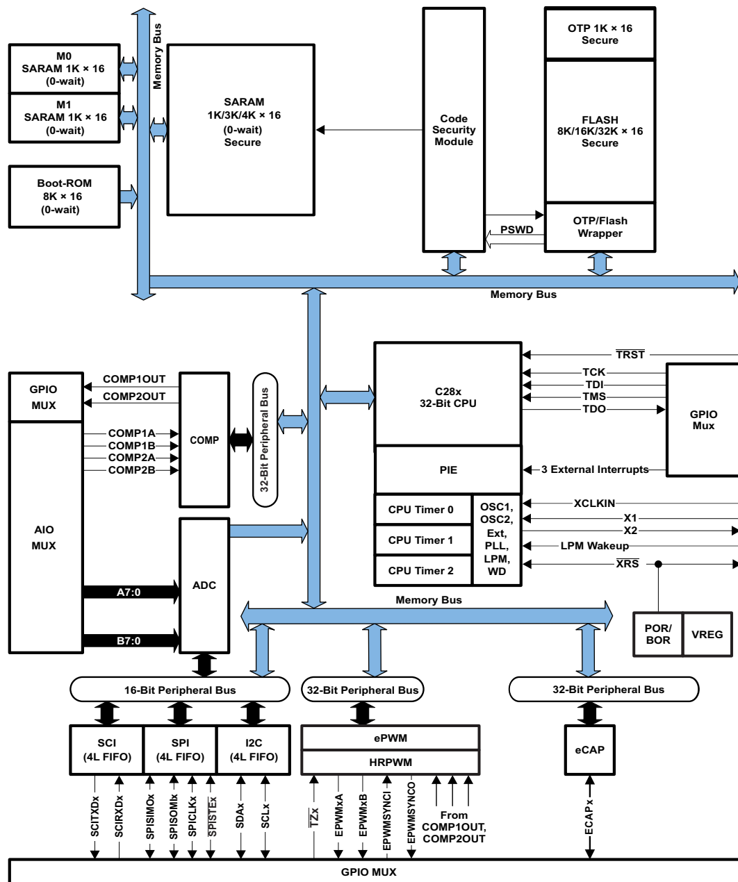
图 1-1. 功能方框图
