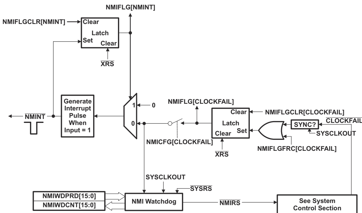
图 8-14. NMI-Watchdog
