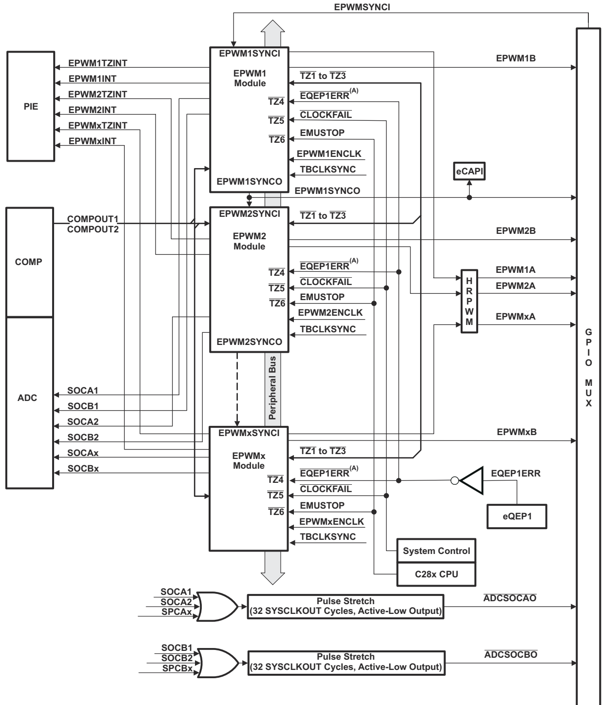
图 8-48. ePWM
