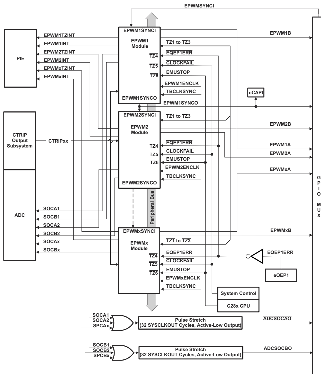
图 8-37. ePWM
