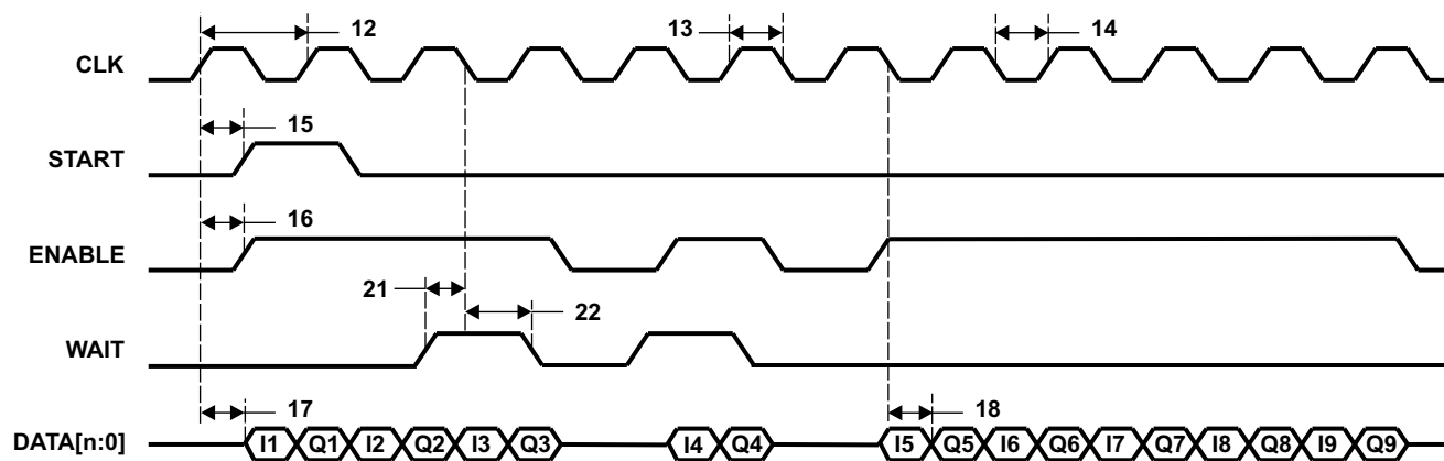
图 8-82. uPP 双倍数据速率 (DDR) 发送时序
