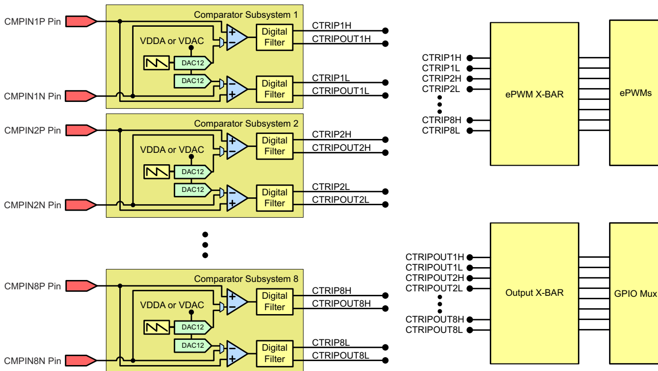
图 8-37. CMPSS 连接 ( 337 焊球 ZWT 和 176 引脚 PTP )
