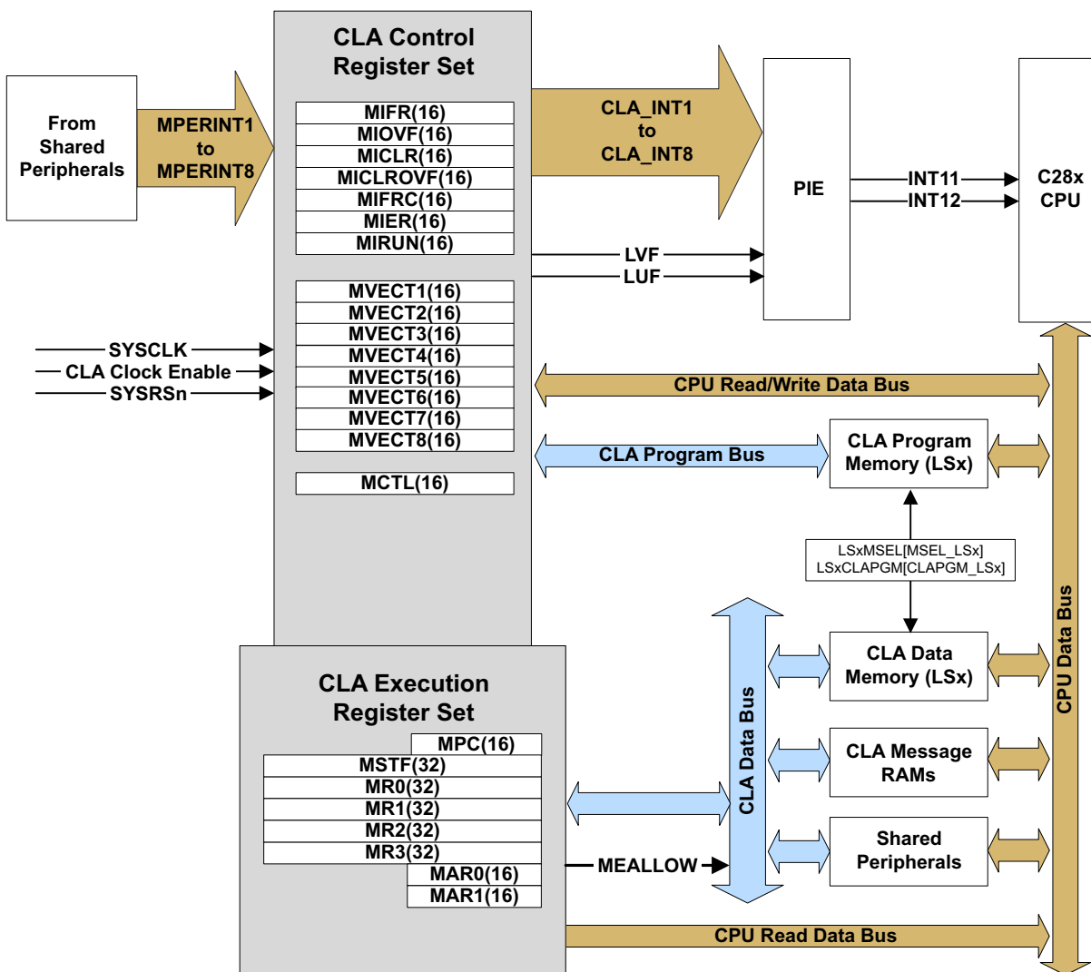
图 9-2. CLA 方框图
