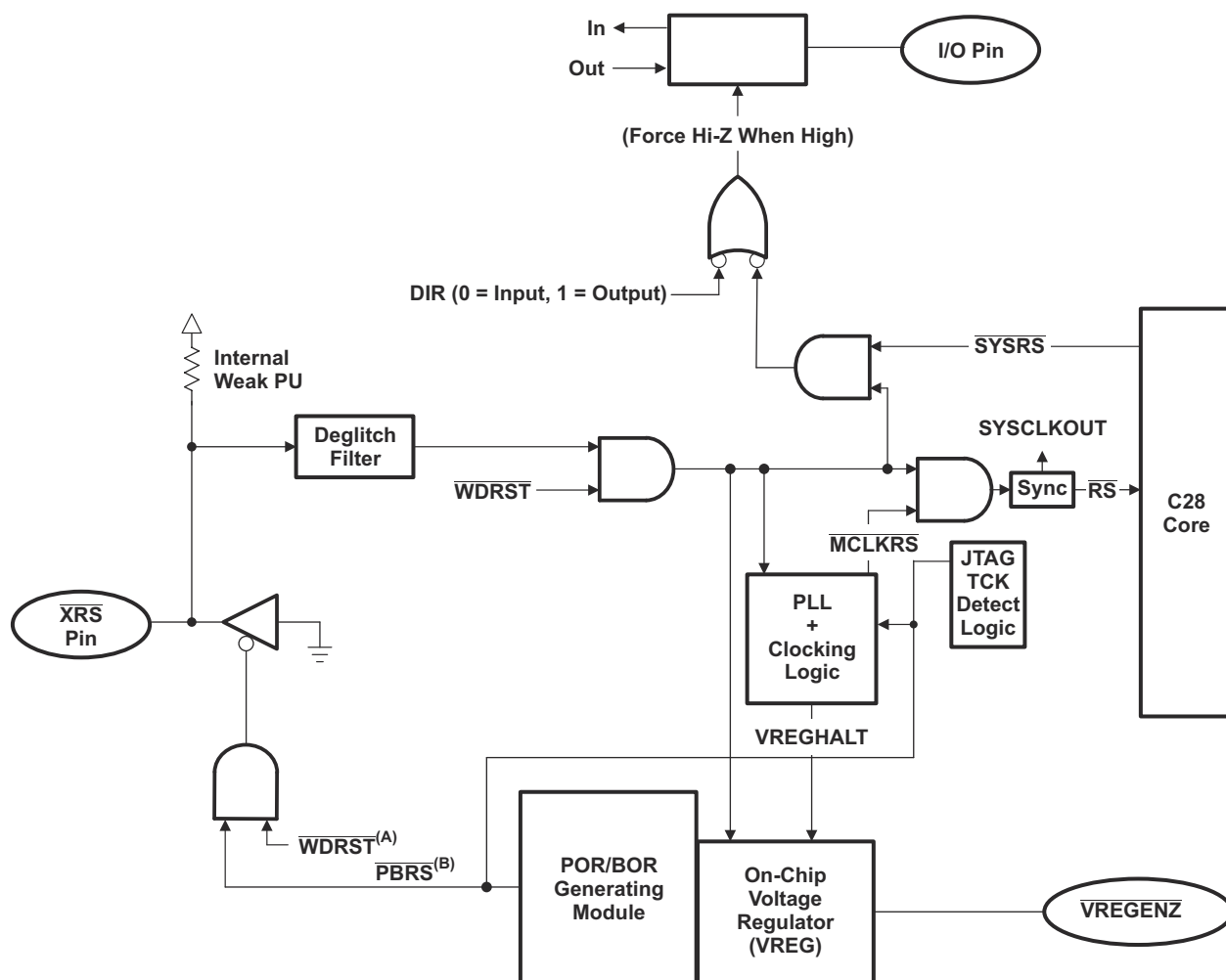
8-9. VREG + POR + BOR + Reset Signal Connectivity
