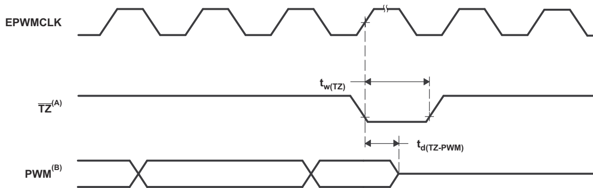
图 7-52. PWM Hi-Z 特性
