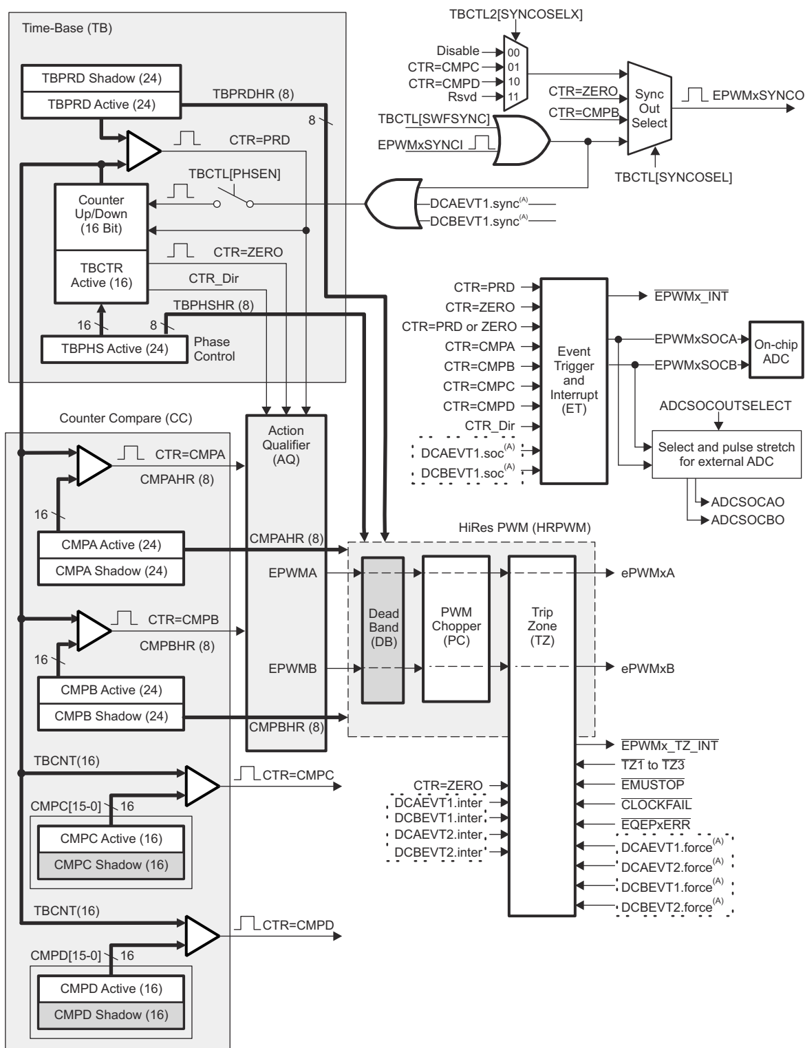
图 7-49. ePWM 子模块和关键内部信号互连
