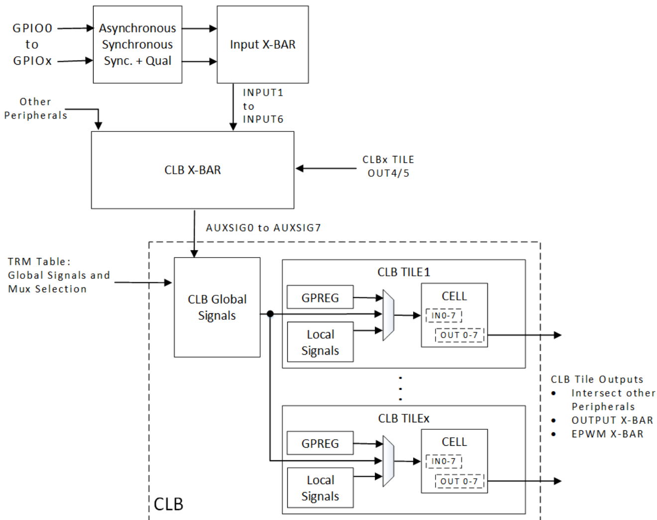
图 6-6. CLB Overview
