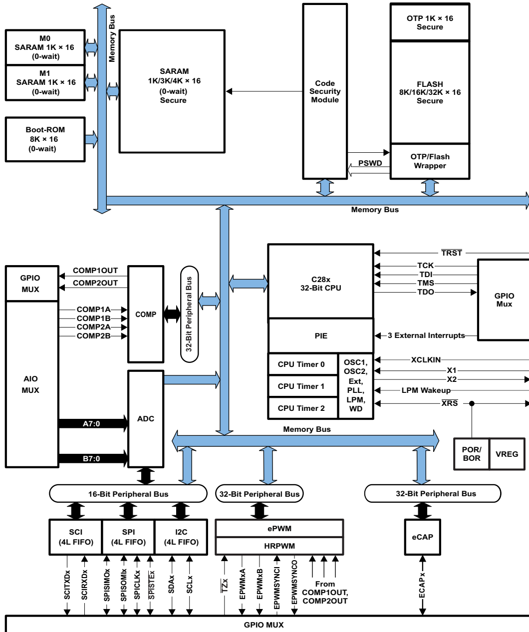
图 1-1. 功能方框图
