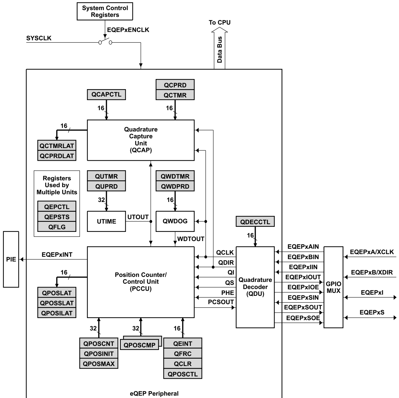
图 7-54. eQEP 方框图
