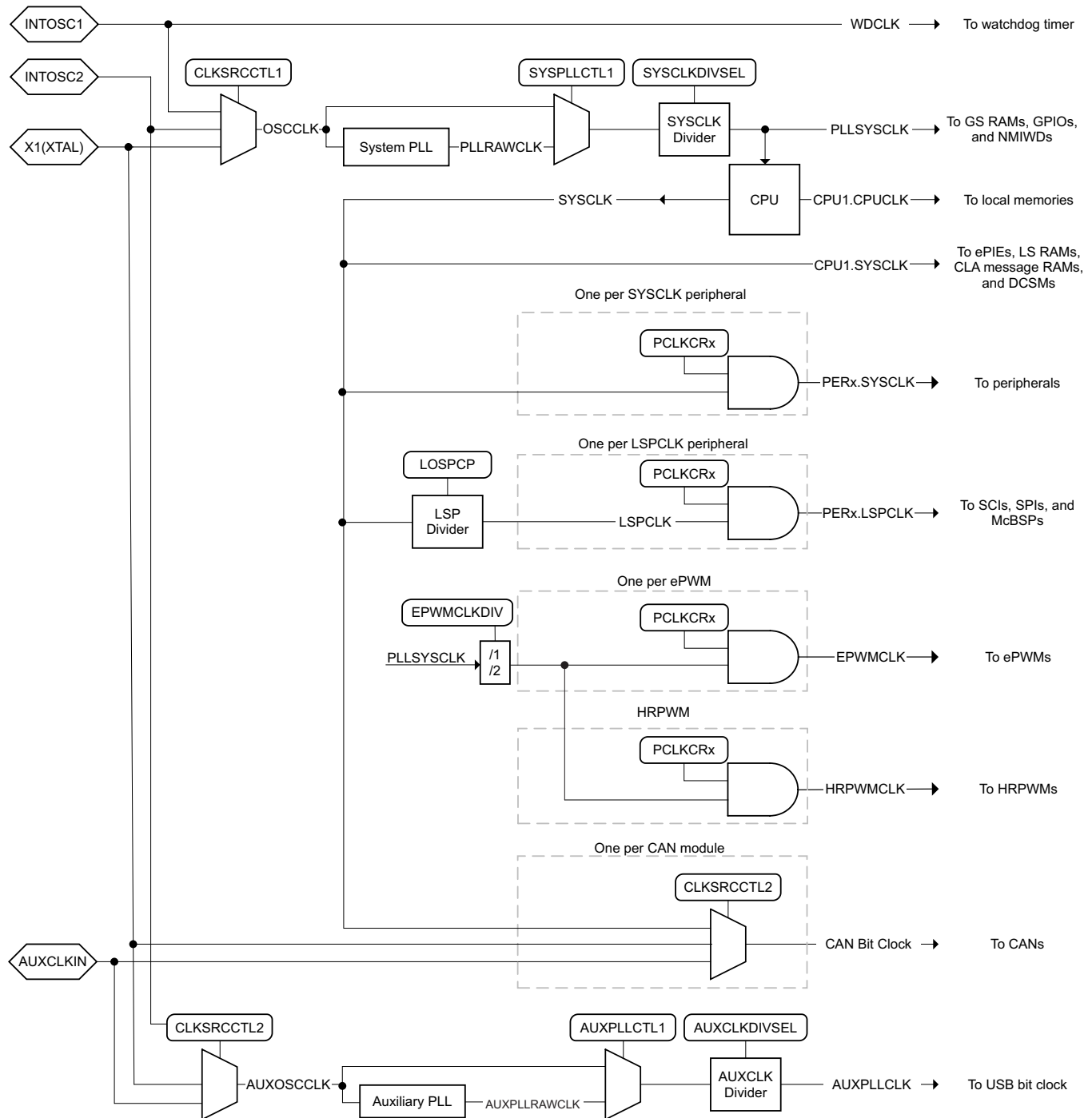
图 5-7. Clocking System
