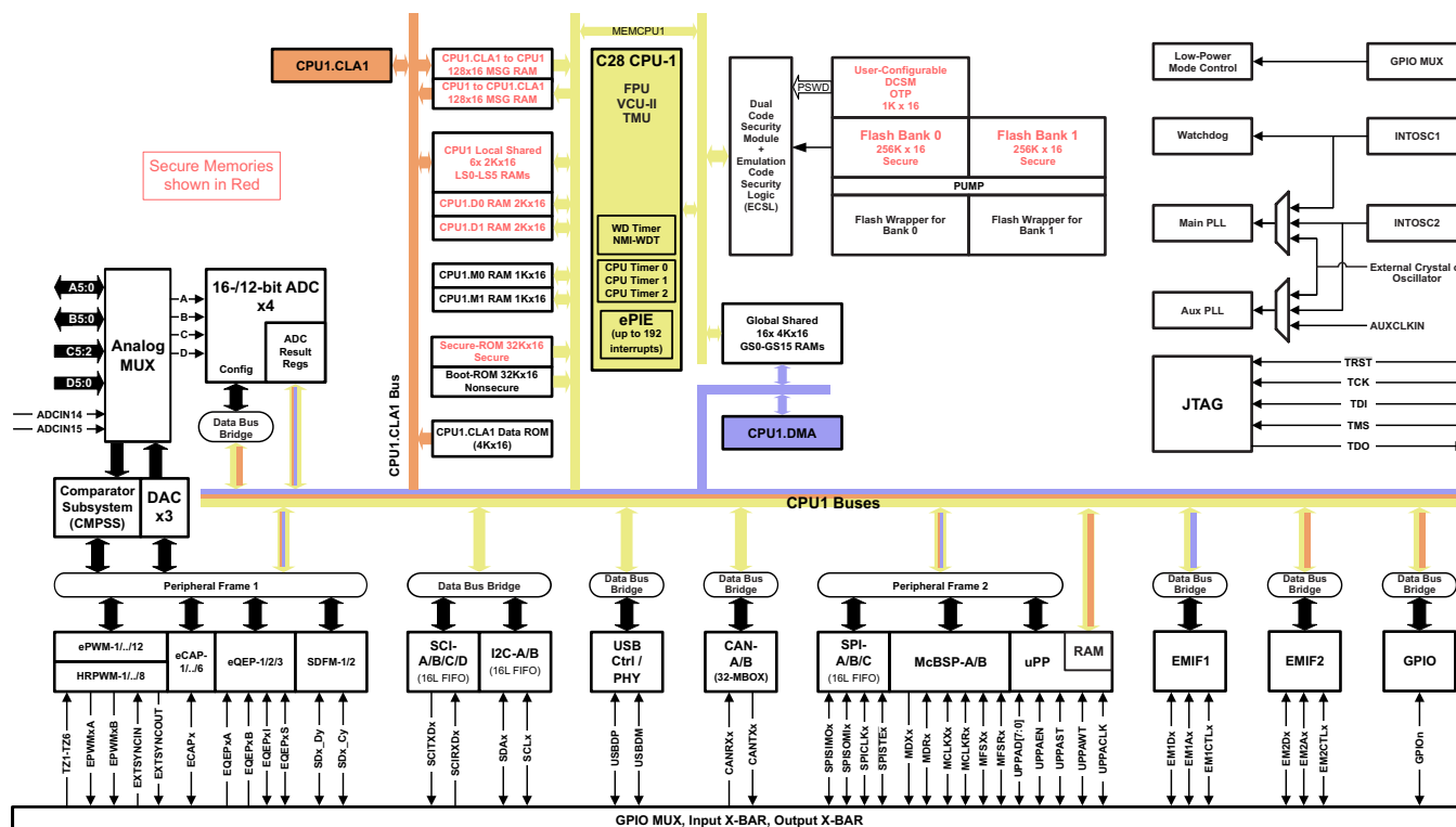
图 1-1. 功能方框图
