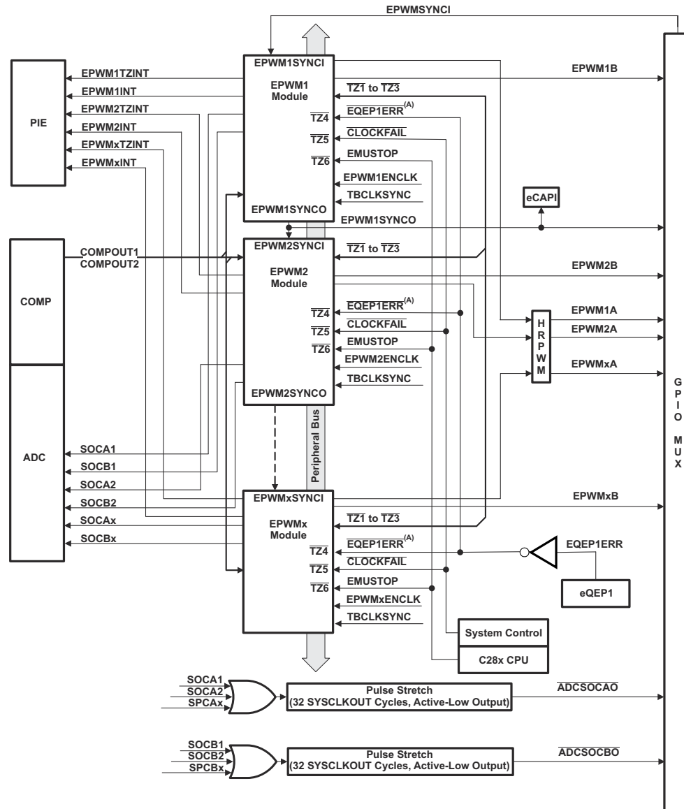
图 8-38. ePWM
