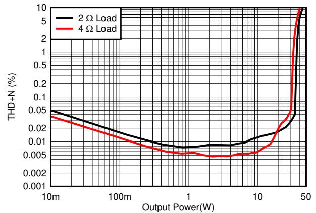
图 6-2. THD+N vs Power - 2 \Omega , 4 \Omega - 18 V
