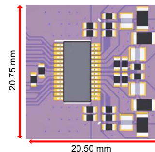
采用铁氧体磁珠的 TPA3138 布局
