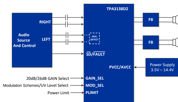
简化原理图
