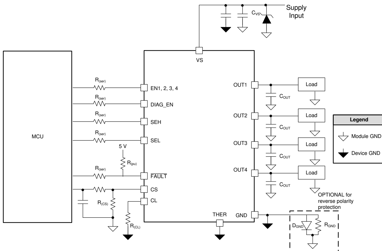
图 9-1. System Diagram
