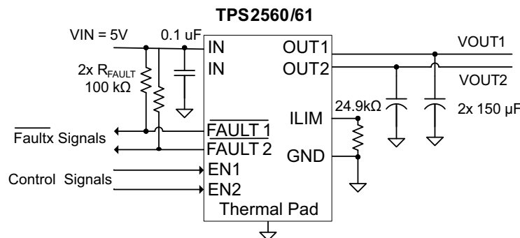
典型应用图
