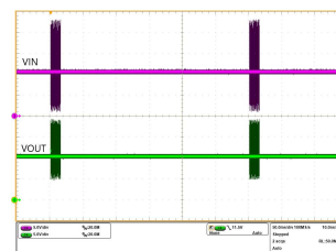
TPS25963x 1KV EFT 响应
