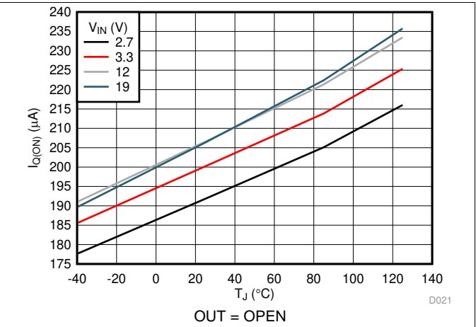
图 3. TPS25962x Quiescent Current
