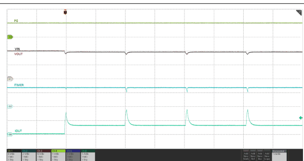
图 9-5. Transient Overload
