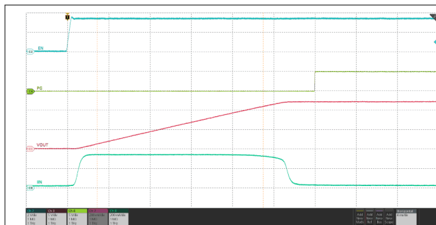
图 9-4. Power Up
