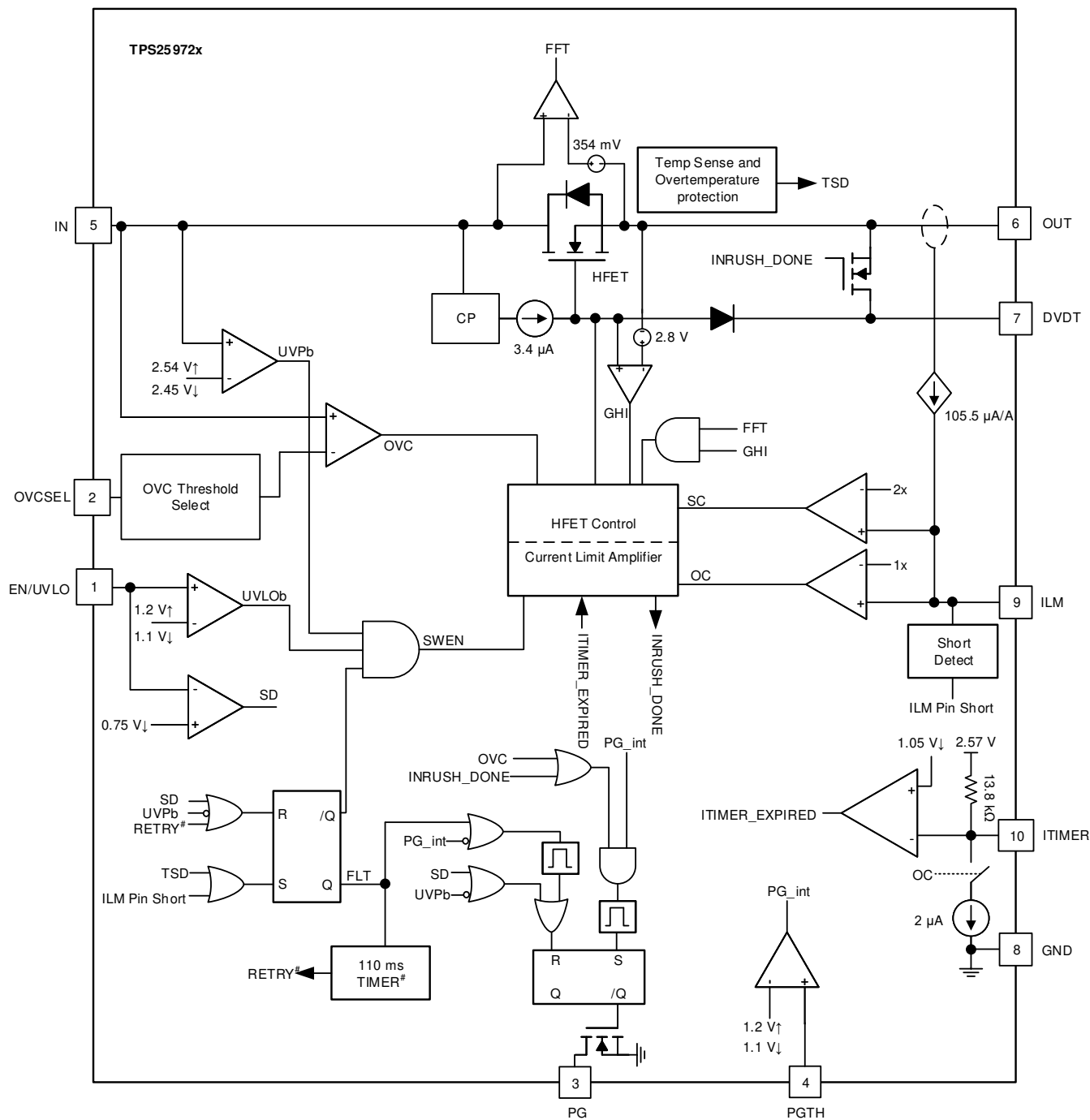
图 8-2. TPS25972x Block Diagram
