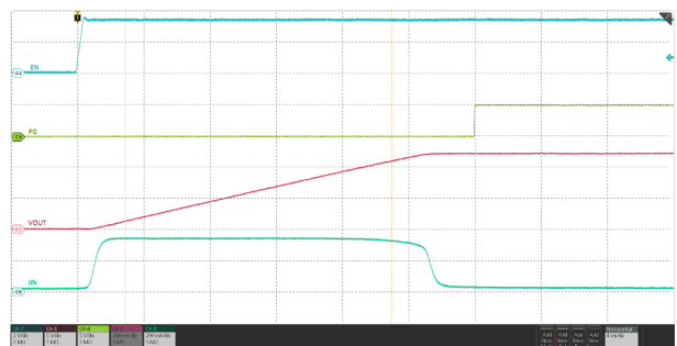
图 7-32. Input Hot-Plug
