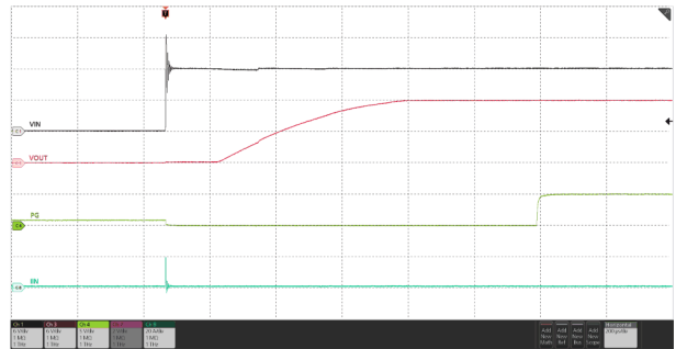
图 7-32. Input Hot-Plug
