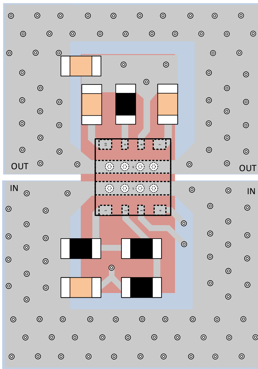
图 11-1. Layout Example
