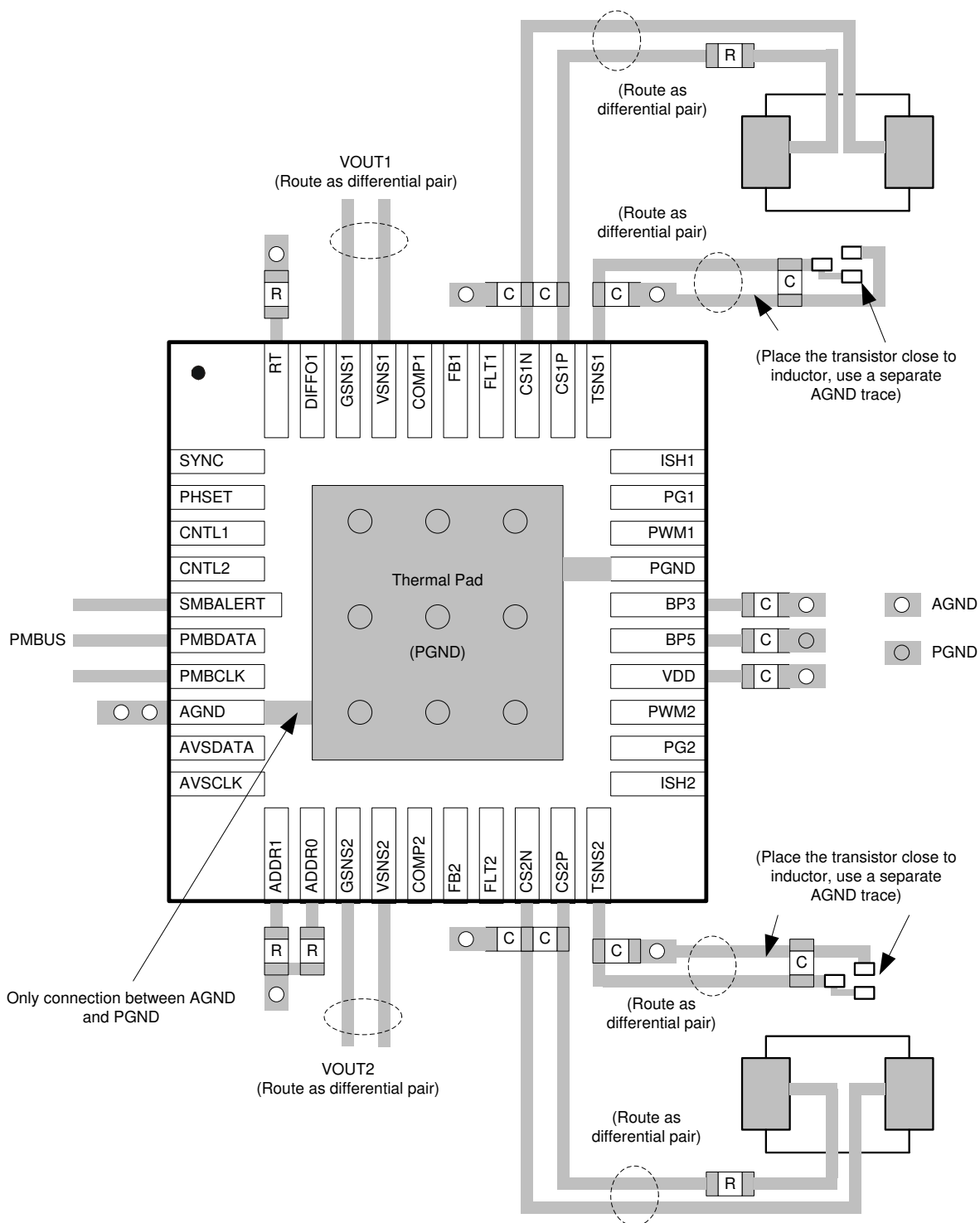
图 34. PCB 布局建议
