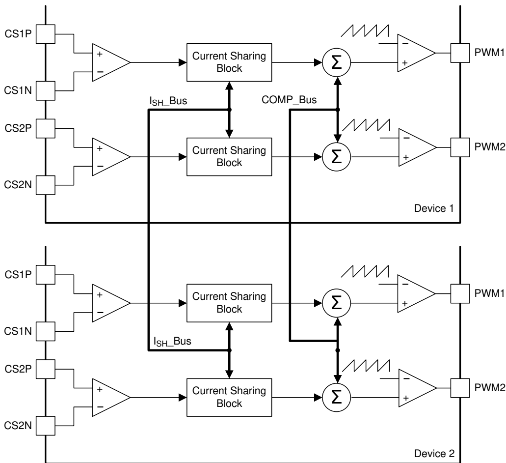
图 18. 电流共享
