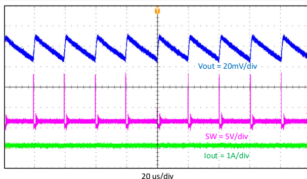
图 9-5. 输出电压纹波, I_{out} = 0.01A
