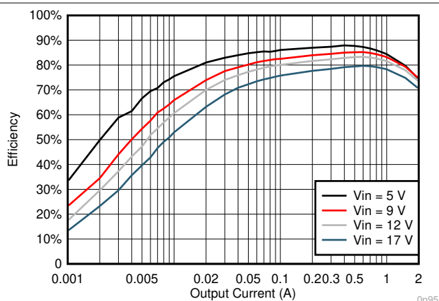
图 7-9. V_{OUT} = 0.95V 效率, L = 2.2\mu H
