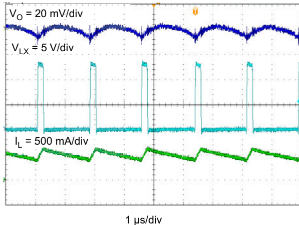
图 8-9. TPS562201 Output Voltage Ripple, I_{OUT} = 2 \text{ A}
