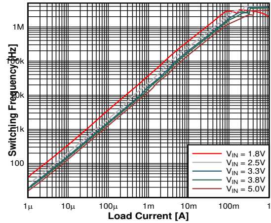
图 9-9. Switching Frequency
