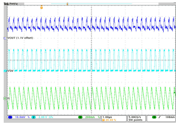
图 9-9. Switching Frequency
