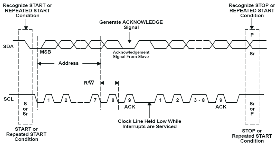
图 8-7. Bus Protocol
