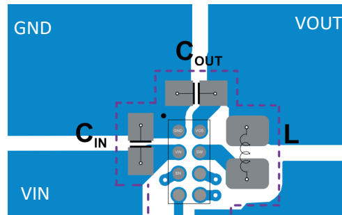
图 11-1. PCB Layout Example
