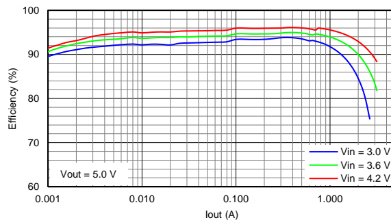
TPS61230 典型应用效率
