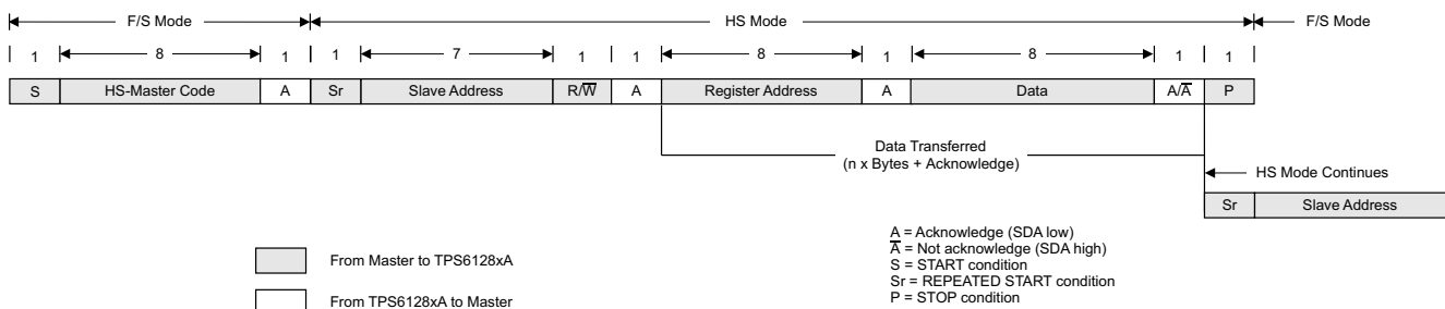
图 26. Data Transfer Format in H/S-Mode
