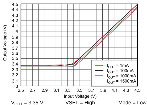
图 38. TPS61281A DC Output Voltage vs Input Voltage
