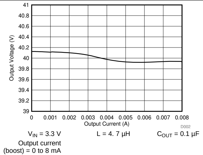
图 2. Load regulation
