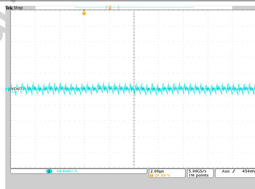
图 10-47. Output Voltage Ripple
