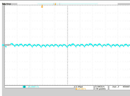
图 10-44. Output Voltage Ripple
