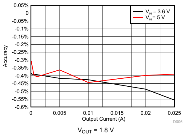
图 7-6. DCDC6 Accuracy
