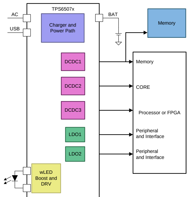
方框图
