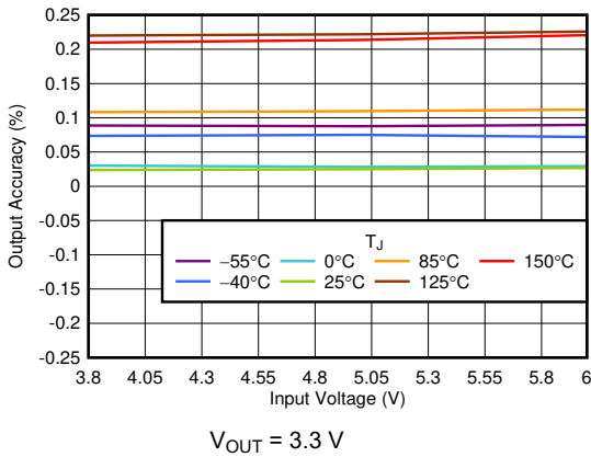
图 6-3. Output Accuracy vs V_{IN}
