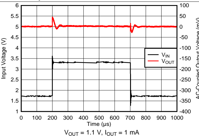
图 14. V_{IN} Transient
