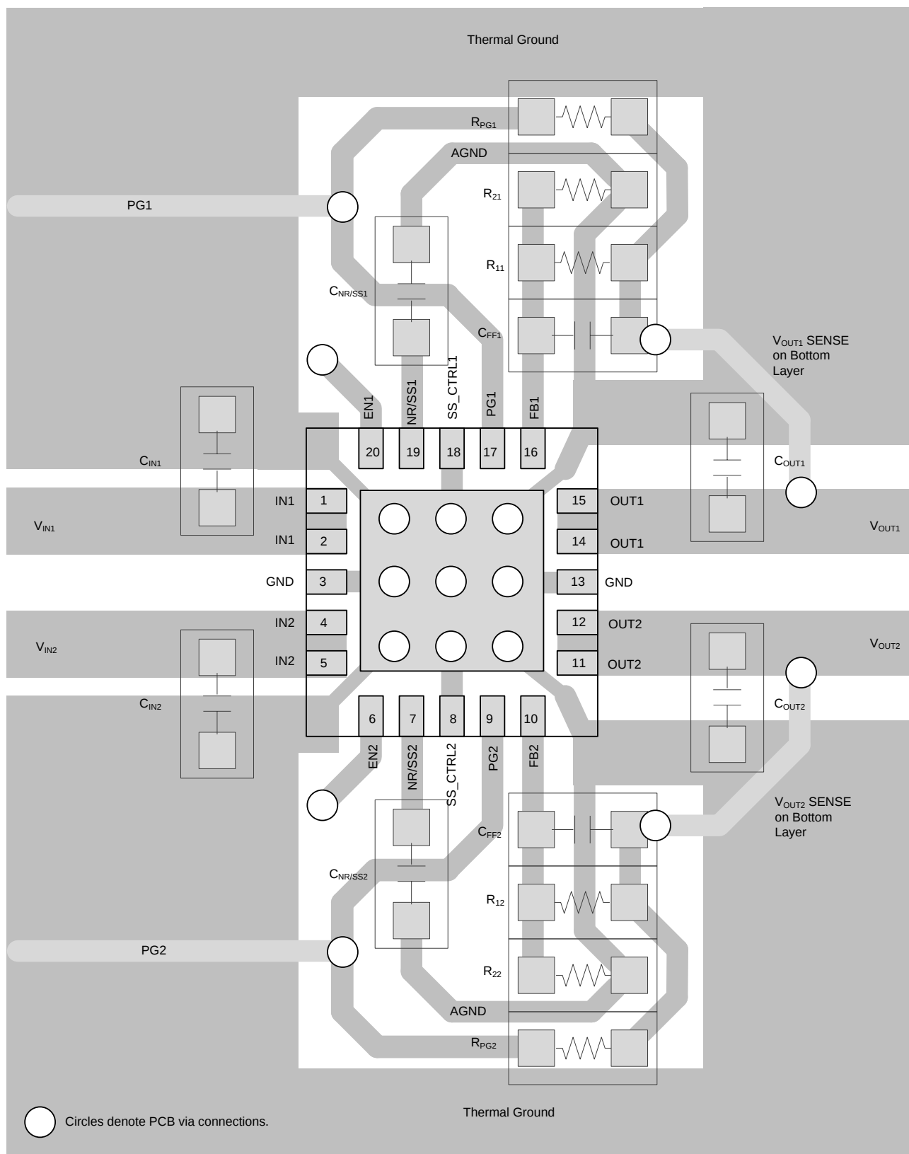
图 65. TPS7A87 Example Layout
