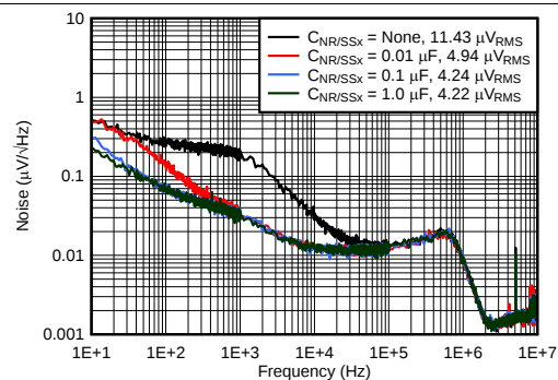
图 8. Output Noise at V_{\text{OUTX}} = 5\text{ V}
