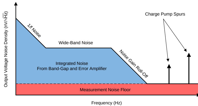
图 49. Output Voltage Noise Diagram
